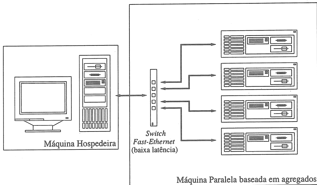
Figura 2: Configuração mínima
