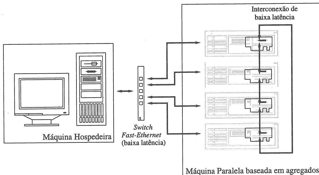
Figura 5: Configuração avançada
