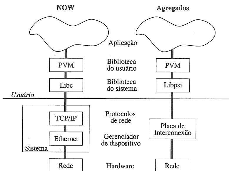
Figura 1: Estrutura de comunicação
