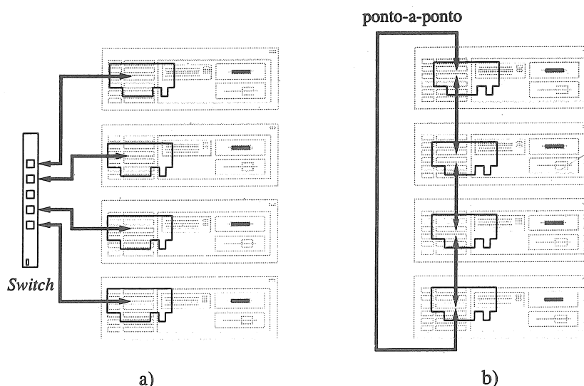
Figura 4: Possíveis formas de interconexão dos nós
